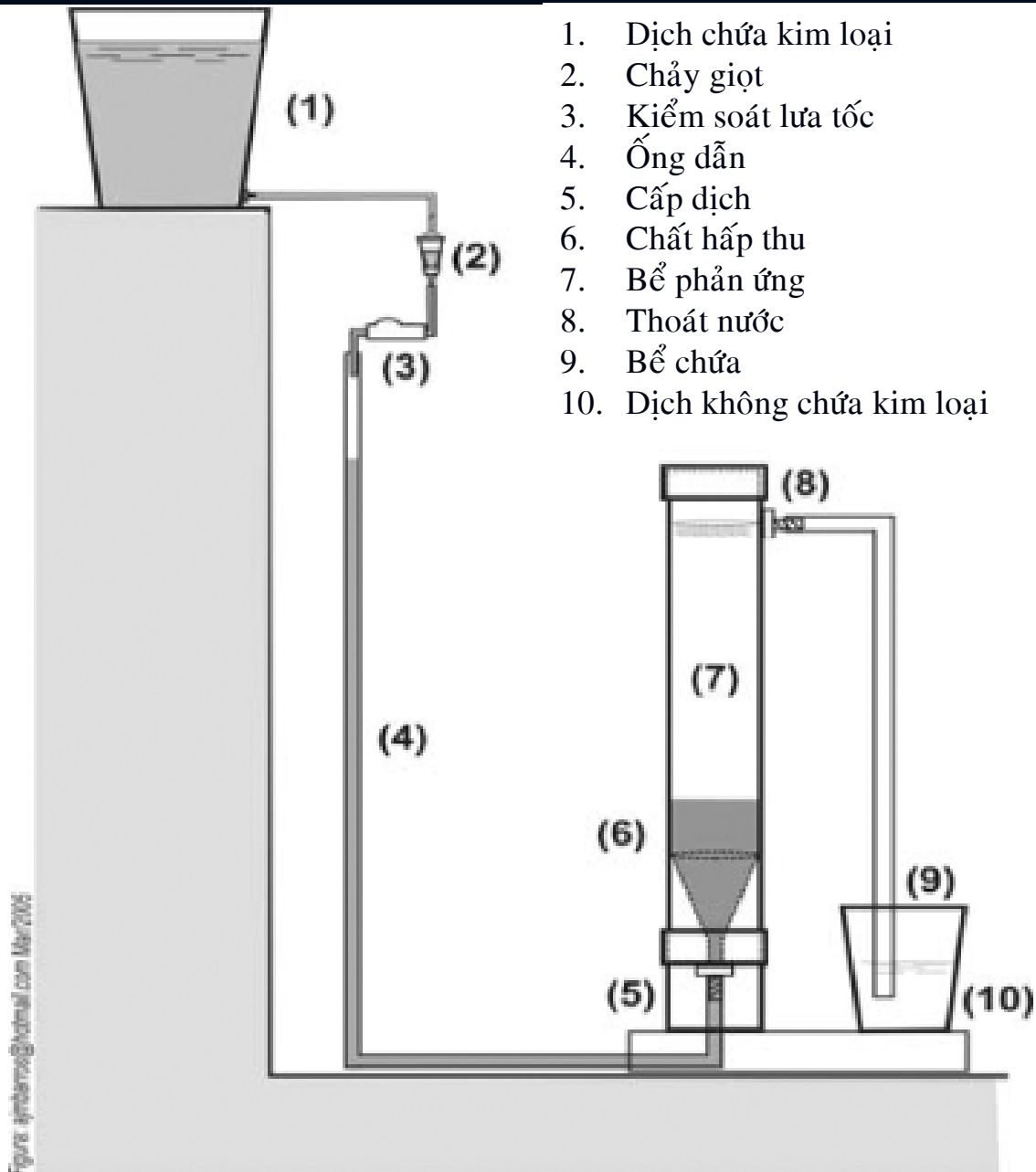
Mô hình phản ứng hấp thu sinh học kim loại
