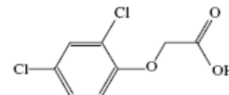
2,4-D
