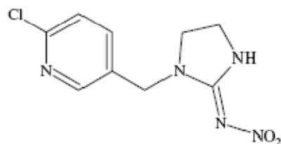
Imidacloprid
